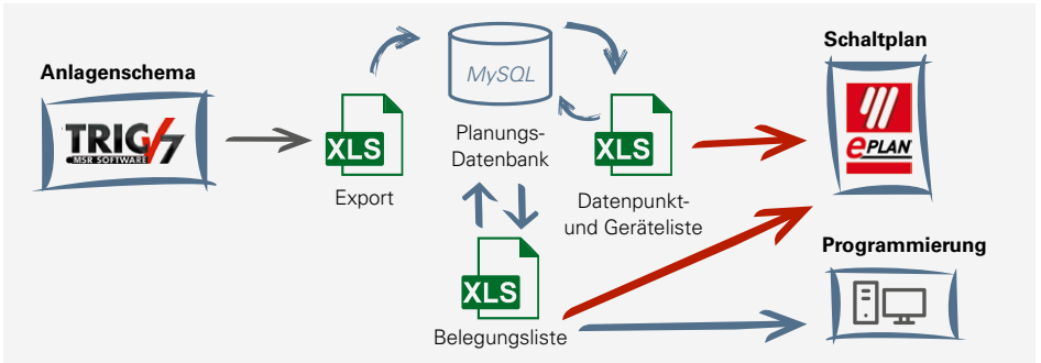
Abbildung 13: Ausschnitt aus dem Planungsablauf – Soll
