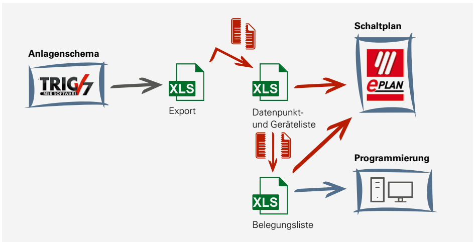
Abbildung 9: Ausschnitt aus dem Planungsprozess – Ist
